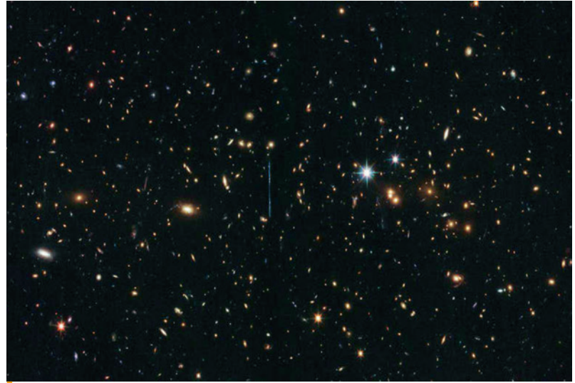
■ Figura 5. La transparencia del universo.
