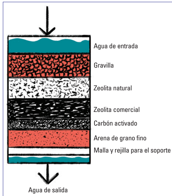
Figura 1. Diseño de un filtro para remover el hierro y manganeso del agua proveniente de pozos de la alcaldía Iztapalapa. Crédito: Diego de la Vega y Judith Cardoso Martínez.
